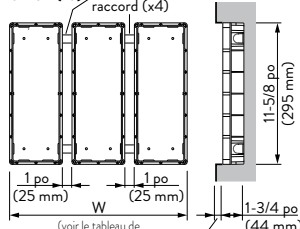
GF-3B (x3) Conduit de raccord (x4)
