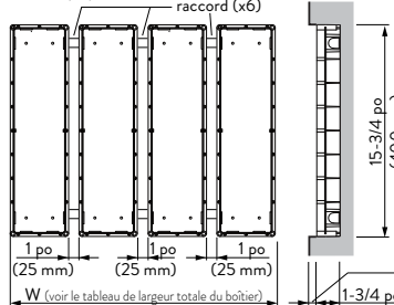
GF-4B (x4) Conduit de raccord (x6)
