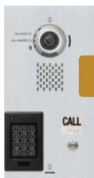
IX-DVF-10KP Poste de porte vidéo IP avec lecteur de proximité Wiegand 125 kHz et clavier d'accès
